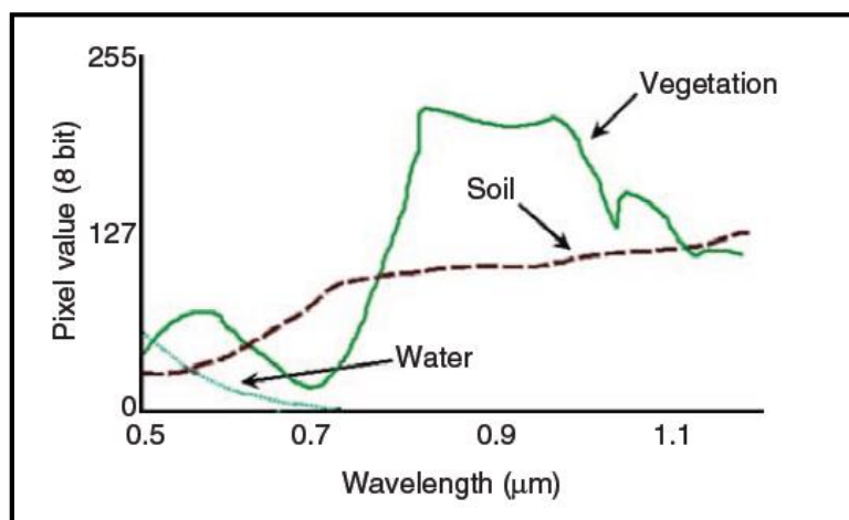
شکل ۲- رفتار طیفی پوشش‌های غالب سطح سیاره زمین
