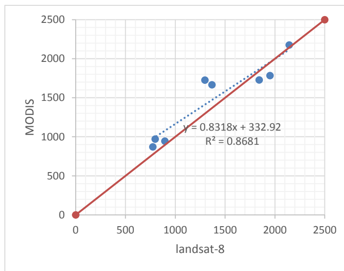
شکل ۴- رابطه رگرسیون خطی مساحت به دست آمده از ماهواره لندست و مادیس (برحسب کیلومتر مربع)
