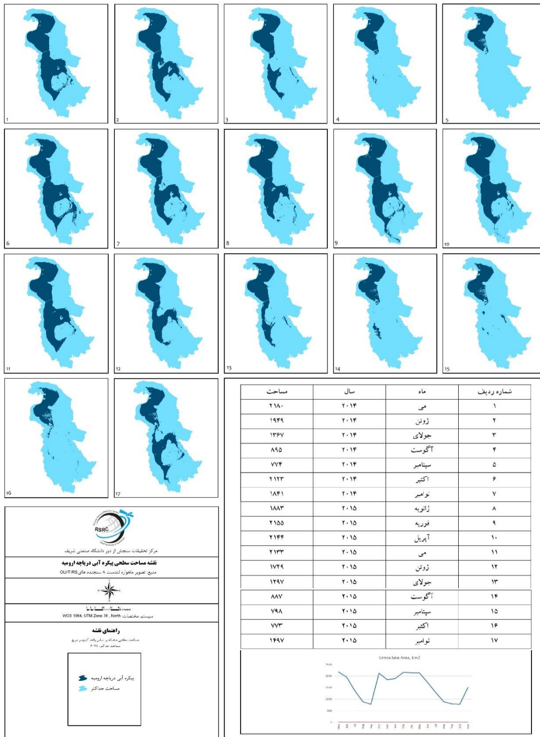
شکل ۱۴- تغییرات ماهیانه مساحت سطحی دریاچه ارومیه نسبت به مساحت حداکثری برای سال‌های ۲۰۱۴ و ۲۰۱۵ میلادی بدست آمده توسط ماهواره لندست ۸
